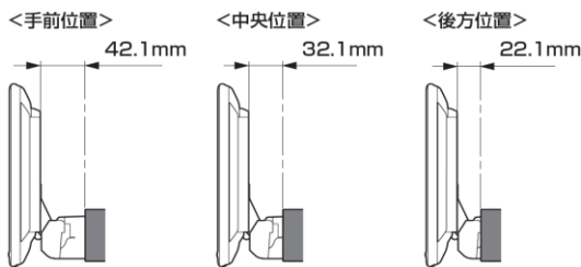
【ディスプレイユニット前後位置】
